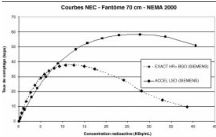
19 Courbes NEC (équivalent de rapport signal sur bruit) mesurées en mode 3D pour différentes catégories d'appareils selon les normes NEMA de 2000. La courbe NEC d'une caméra équipée de LSO (courbe ACCEL LSO) atteint son maximum pour une concentration plus élevée que celle correspondant au maximum de la courbe d'une caméra BGO (courbe EXACT HR+ BGO). L'amélioration des performances en taux de comptage apportée par des nouveaux scintillateurs plus rapides, tels que le LSO, permet de réduire la durée des acquisitions tout en conservant une statistique suffisante pour l'obtention d'une image de qualité.
