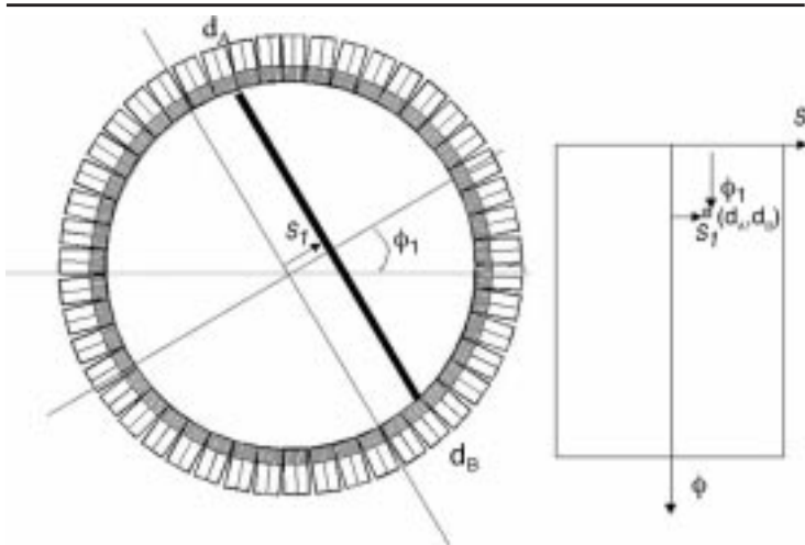
6 Acquisition des données. Une ligne de réponse entre deux détecteurs d_A et d_B est définie dans le repère des projections par son angle ( \varphi_1 ) et sa distance par rapport au centre du tomographe ( s_1 ). La mesure d'une ligne de réponse incrémentée d'une unité le pixel du sinogramme correspondant à l'angle et à la distance par rapport au centre.
