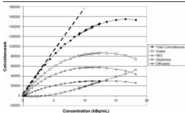
17 Performances en taux de comptage de la caméra C-PET ® (Adac-Philips).
