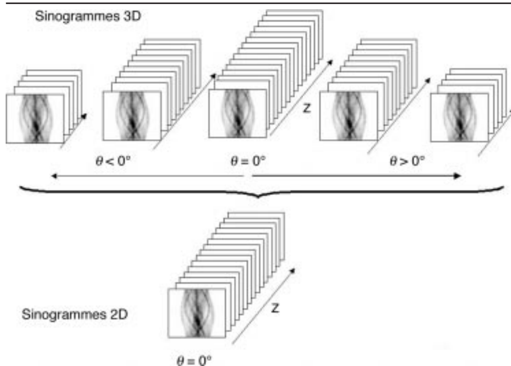
13 Principes des algorithmes de réarrangement des données. Le but des algorithmes de réarrangement des données consiste à convertir une série de sinogrammes mesurés en mode 3D pour des angles \theta différents en un ensemble de sinogrammes correspondant à des angles \theta = 0^\circ . Les sinogrammes 2D obtenus peuvent être reconstruits par des techniques de reconstruction bidimensionnelle rapides.
