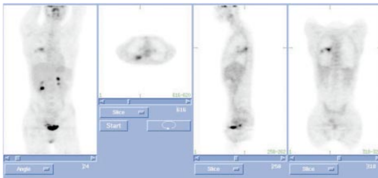
20 Analyse dans les trois plans de coupe d'un examen FDG en mode corps entier acquis par le C-PET ® en émission/transmission en 1 heure. L'image de la projection calculée fournit une représentation volumique de la distribution du traceur (Hôpital d'Instruction des Armées du Val de Grâce. C-PET ® . Adac-Philips). Illustration clinique à partir d'un cas de masse tumorale maligne pulmonaire postérieure droite.
