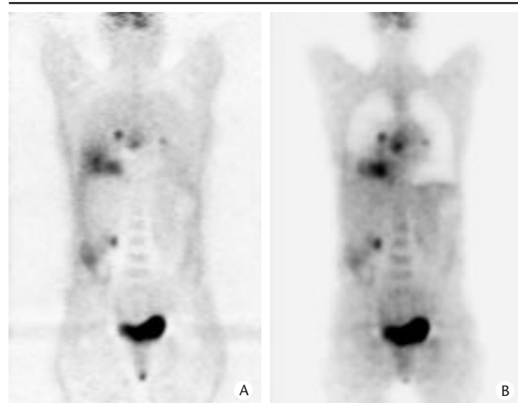
14 Impact de la correction d'atténuation en pratique clinique. A. Coupe coronale sans correction d'atténuation. B. Coupe coronale avec correction d'atténuation. La correction d'atténuation permet une meilleure visualisation des structures profondes (rachis), et facilite la localisation des différentes lésions. Illustration clinique : tumeur maligne basipulmonaire droite, avec extension hilaire bilatérale et médiastinale précarinaire (Hôpital d'Instruction des Armées du Val de Grâce. C-PET ® . Adac-Philips).
