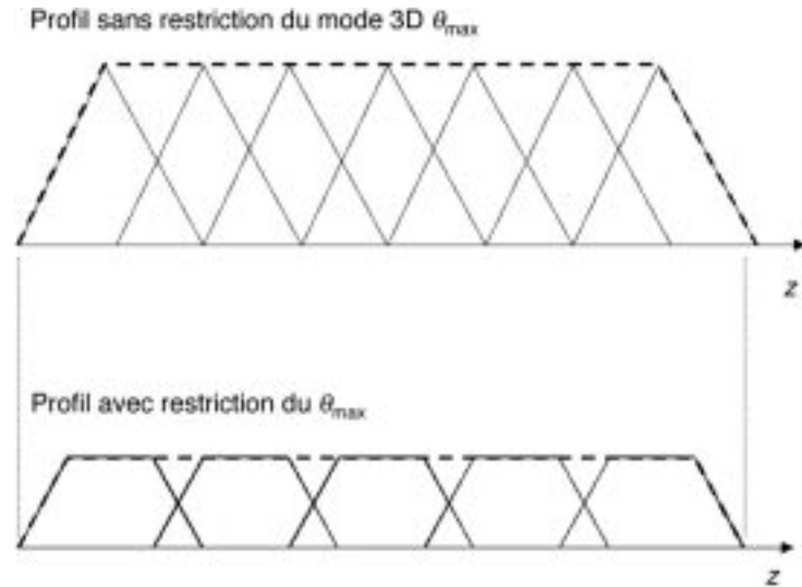
11 Influence de l'angle d'ouverture ( \theta ) du mode d'acquisition 3D sur la réalisation des examens corps entier. Une réduction de l'angle d'acceptance entraîne une diminution de la sensibilité (restriction du \theta_{max} ), mais permet de couvrir un champ de vue axial avec moins de pas successifs par rapport à une mesure sans limitation d'angle.
