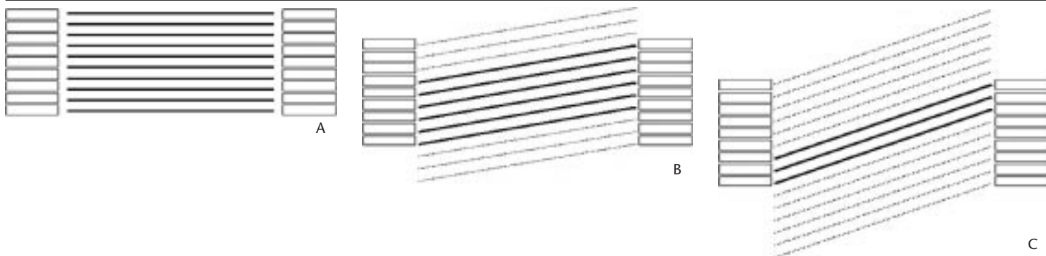
12 Sinogrammes en mode 3D et projections incomplètes. A. Sinogrammes correspondant à une incidence identique au plan des détecteurs correspondant à un angle \theta = 0^\circ , donc identiques au mode d'acquisition 2D. B. Sinogrammes correspondant à une différence de trois couronnes de détecteurs
