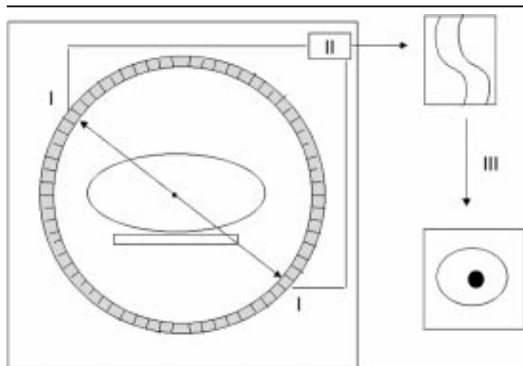
2 Les différents modules d'un tomographe à émission de positons. La formation de l'image résulte de la détection des deux photons \gamma de 511 keV émis lors de la réaction d'annihilation. Pour y parvenir, des détecteurs élémentaires sont répartis en anneau autour du patient (I). Le circuit électronique accepte la coïncidence si les deux événements arrivent dans une fenêtre temporelle de l'ordre de 10 ns, et si les deux photons ont une énergie voisine de 511 keV (II). La dernière étape (III) est constituée par la reconstruction des données, permettant d'obtenir l'image de la distribution radioactive au sein du patient.
