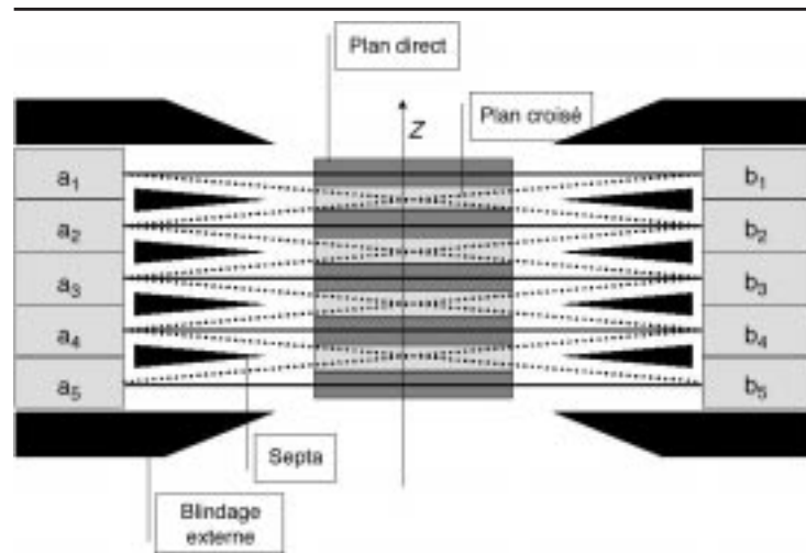
7 Principe du mode d'acquisition 2D. Les plans directs sont reconstruits à partir des lignes de réponse mesurées au sein d'une couronne de détecteurs (par exemple entre a_1 et b_1 ). Les plans croisés sont constitués des lignes de réponse entre deux couronnes jointives (par exemple entre a_1 et b_2 ). Les lignes de réponse entre des couronnes non jointives ne sont pas mesurées (par exemple entre a_1 et b_3 ) du fait de la présence des septas.
