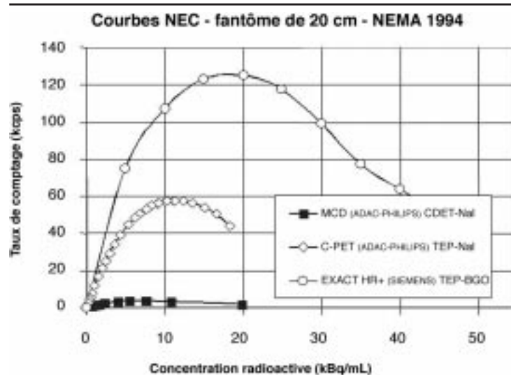
18 Courbes NEC (équivalent de rapport signal sur bruit) mesurées en mode 3D pour différentes catégories d'appareils selon les normes NEMA de 1994. Les faibles performances des gamma-caméras en coïncidence s'expliquent par l'utilisation d'un cristal de NaI(Tl) d'une épaisseur inférieure à 19 mm, et par un angle solide de détection assez réduit (courbe MCD – CDET). Les TEP équipés de six détecteurs de NaI(Tl), répartis en anneau autour du patient, entraînent une augmentation du maximum de la courbe NEC d'un facteur 10 par rapport aux systèmes précédents (courbe C-PET TEP-NaI). Le phénomène de saturation, pour les systèmes constitués de détecteurs plans de NaI(Tl), se produit pour des concentrations relativement faibles, en raison de la grande surface de détection. Les TEP conçus à partir de détecteurs blocs sont moins sensibles aux phénomènes d'empilement. De plus, la forte densité du cristal BGO (germanate de bismuth) permet d'obtenir des performances en taux de comptage supérieures aux systèmes NaI(Tl) (courbe EXACT HR+ BGO).
