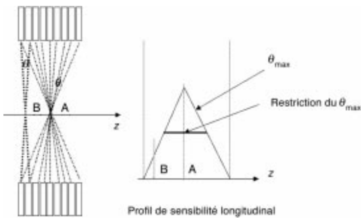
10 Variation de la sensibilité, en mode 3D, dans la direction longitudinale. L'angle \theta correspond à l'angle d'incidence d'une ligne de réponse par rapport au plan perpendiculaire au détecteur. Cet angle est de 0^\circ en mode 2D. En revanche en mode 3D, cet angle dépend de la position des détecteurs sur des couronnes différentes. Une source positionnée au centre du tomographe (A) est vue avec un angle solide plus important qu'une source excentrée (B). Il en résulte une variation longitudinale de la sensibilité, en fonction de la position de la source. Lorsque l'angle d'acceptance est limité, le profil de sensibilité se transforme en un trapèze.
